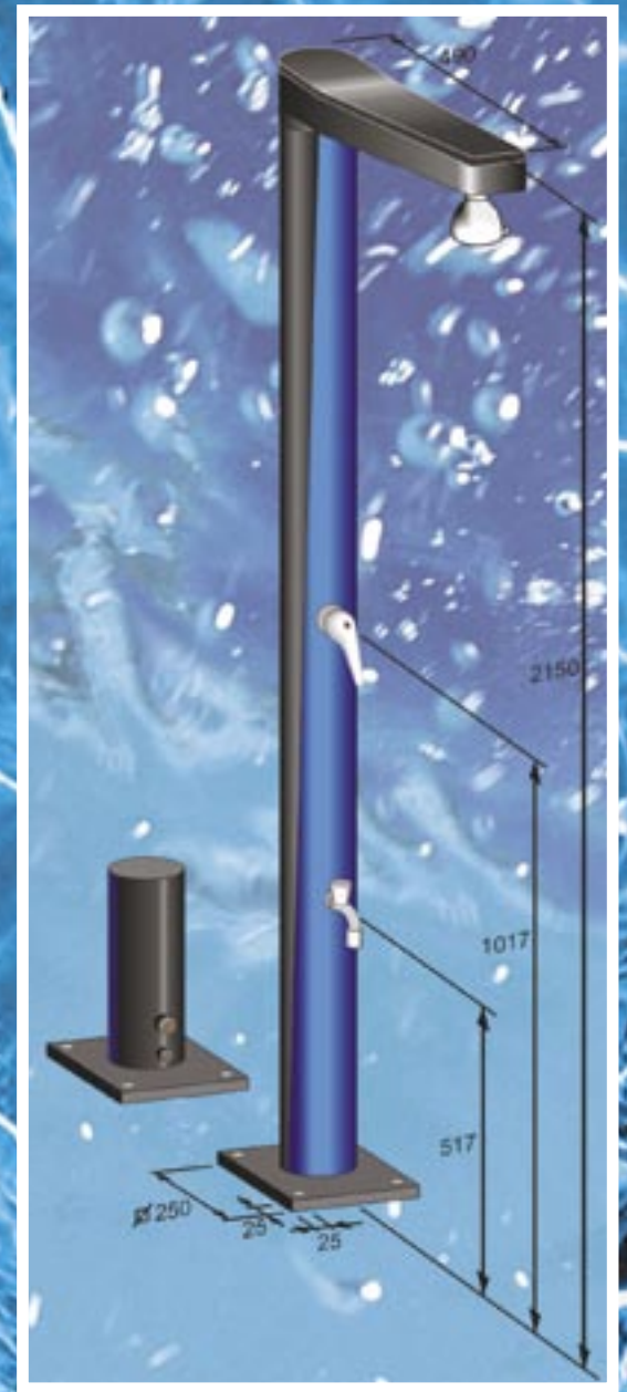
Vakaa asennusalusta ja käytännöllinen venttiili pylvään talvityhjennykseen
